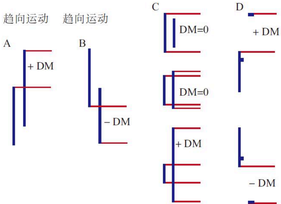
图24-1 趋向运动
